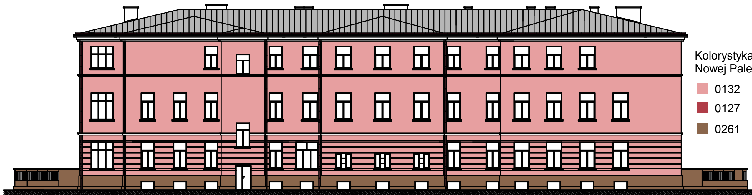
Elewacja tylna północna 1 : 100
